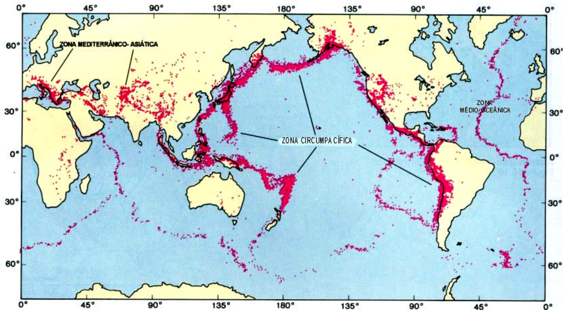
Fig.25 – Distribuição mundial de sismos e localização das três grandes zonas sísmicas (modificado de Skinner & Porter, 1987).
