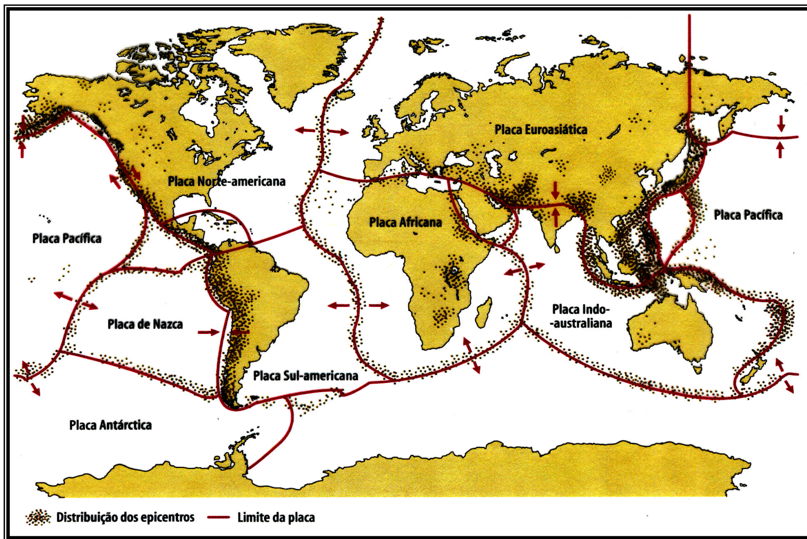
Fig.27 – Distribuição dos sismos no mundo (adaptado de transparências Areal Editores).
