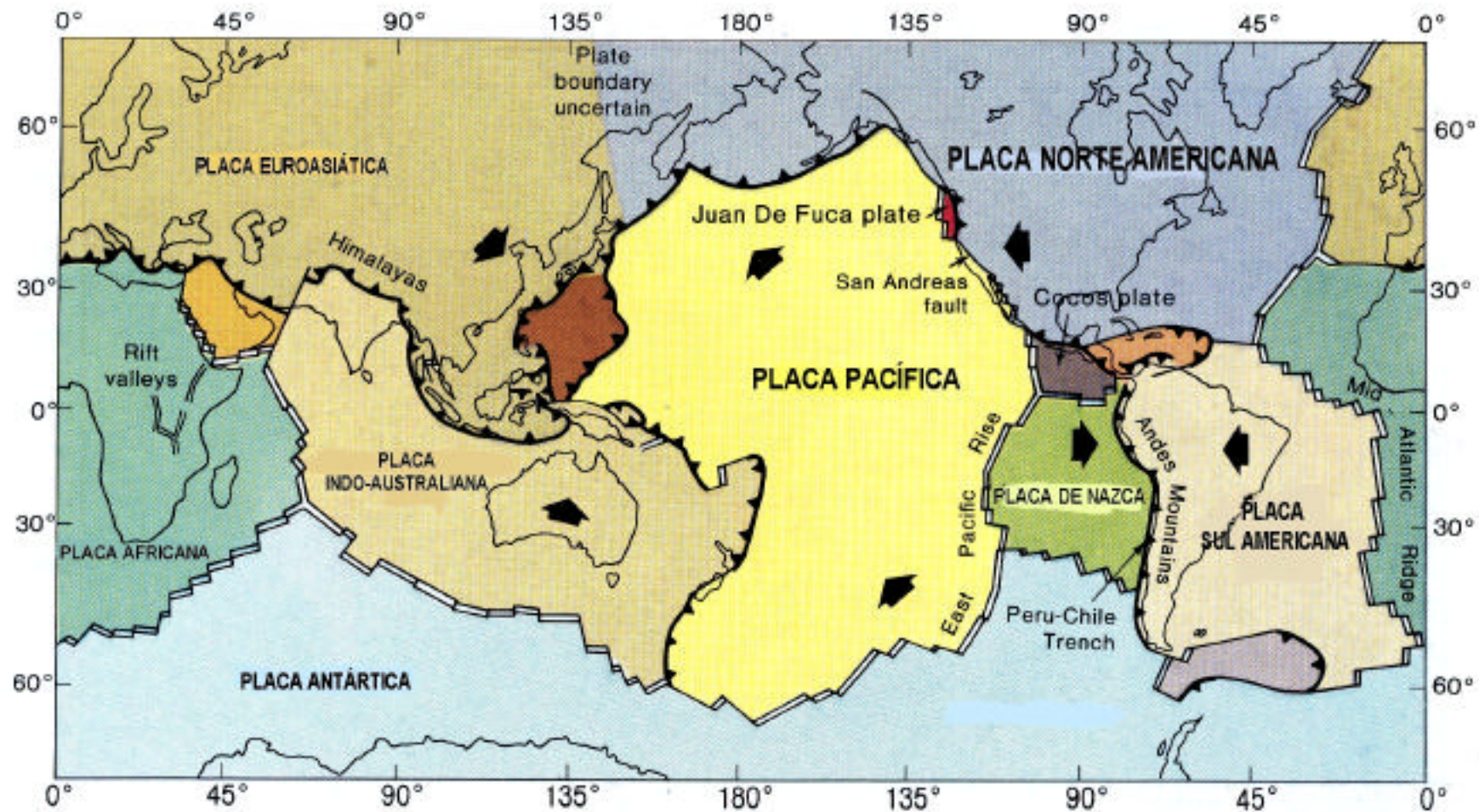
Fig. 26 - Maiores placas tectónicas do Mundo (modificado de Skinner & Porter, 1987).
